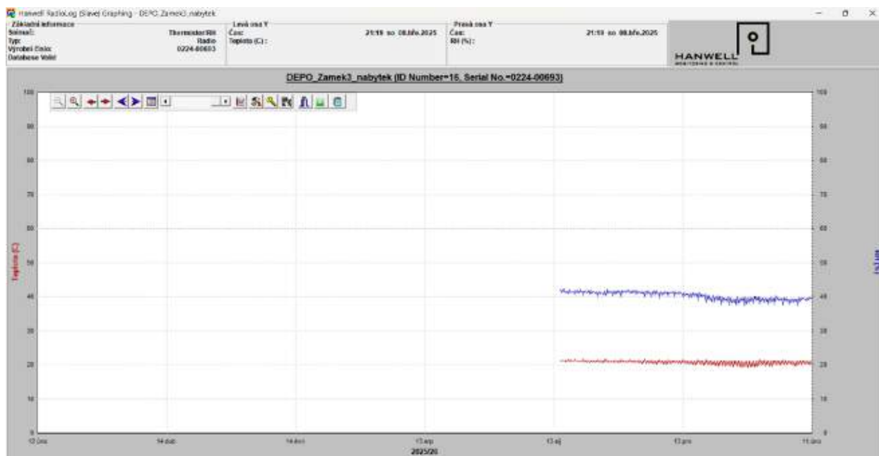
Obr. 4: Ukázka nově nainstalovaného čidla a křivky měření RV/T v místnosti depozitáře podsírký B, v budově Zámek 3 za rok 2025.
