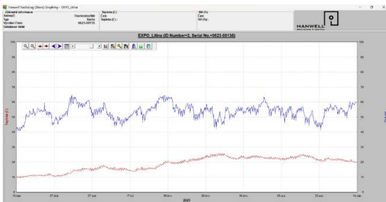
Obr. 5: Ukázka ročních křivek RV/T v jedné z místností expozice Blanenská umělecká litina za rok 2025.
