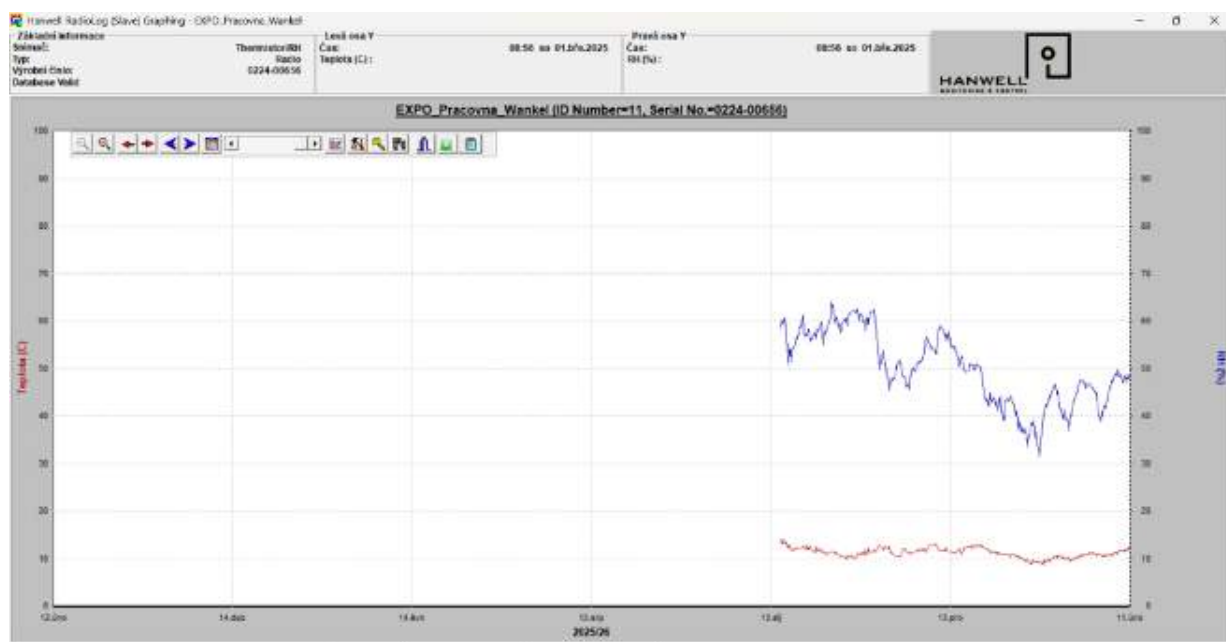
Obr. 3: Ukázka nově nainstalovaného čidla a křivky měření RV/T v místnosti expozice Obrazy z Moravského Švýcarska v období za rok 2025.
